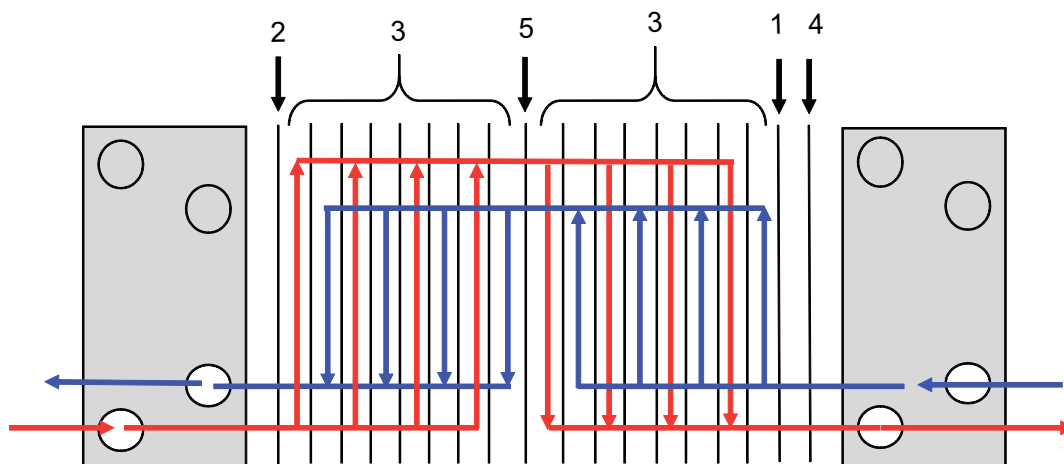
3. ábra: Példa a többjáratos kialakításra.
