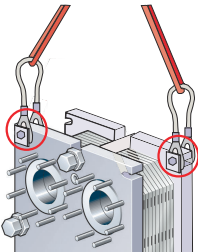
8. ábra: A AQ4T, AQ2T, AQ3, AQ2L emelése
