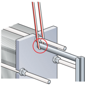
6. ábra: Az AQ1, AQ2, AQ4, AQ1A, AQ2A, AQ1L és a AQ3, AQ2L régi verziójának emelése
