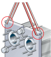
5. ábra: Az AQ1, AQ2, AQ4, AQ1A, AQ2A, AQ2S, AQ1L és a AQ3, AQ2L régi verziójának emelése
