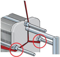
7. ábra: Az AQ2S emelése.
