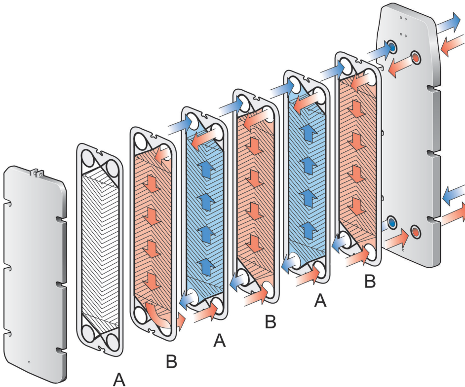
Figure 2 : Principe d'agencement de jeu de plaques, joints face au bâti mobile.
