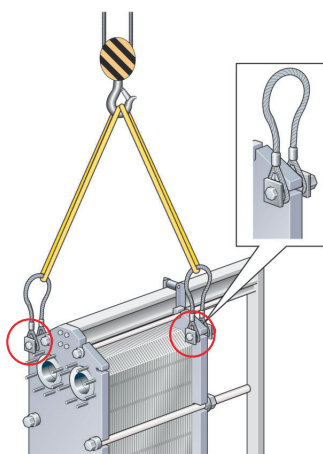
Figura 5: Dispozitiv de ridicare pentru M15, TL10, TL15, T20, TS20, WideGap 100 și WideGap 200.
