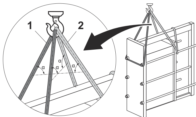
Figura 4: Ilustrația arată modul de înfiletare a chingilor de troliu.
