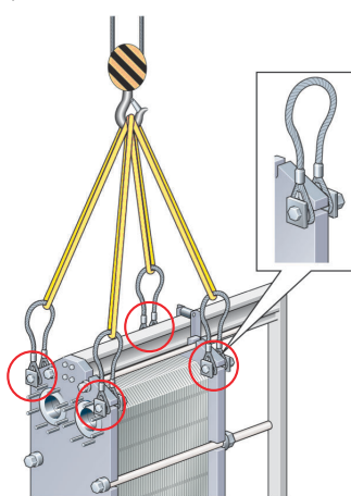
Figura 6: Dispozitiv de ridicare pentru T25, MX25 și MA30-S.
