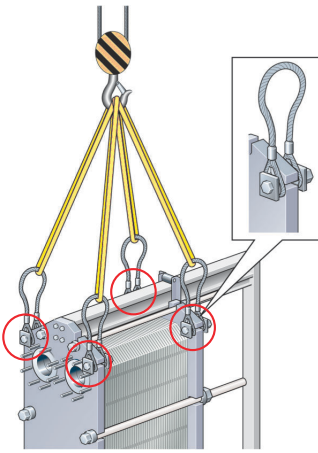
Σχήμα 5: Διάταξη ανύψωσης για AQ10T και AQ10.
