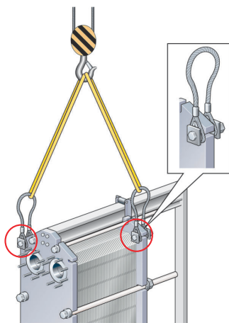
Σχήμα 4: Διάταξη ανύψωσης για AQ6, AQ4L, AQ6L, AQ8 και AQ8S.
