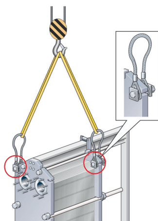
4. attēls: Celšanas ierīce, paredzēta AQ6, AQ4L, AQ6L, AQ8 un AQ8S.
